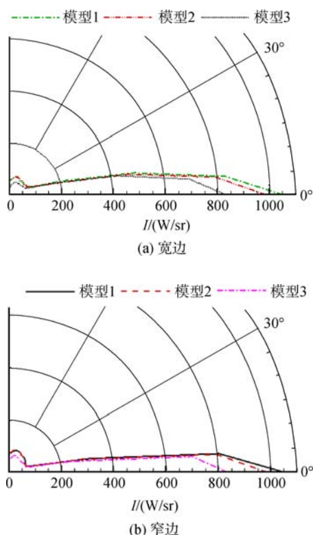
图10 不同方位角下的红外辐射强度分布图
