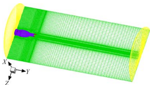
图 3 模型 3 计算域整体网格
