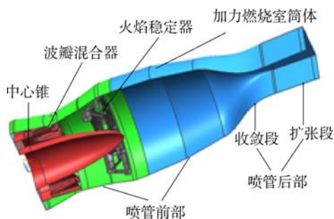
图 1 圆转矩形喷管
