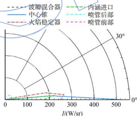
图9 高温部件红外辐射强度分布(模型1)
