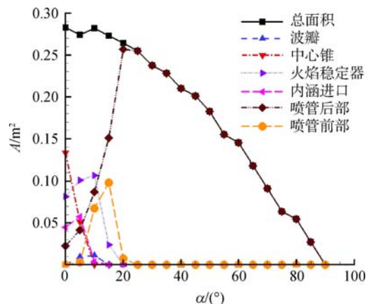
图7 固体壁面探测面积随方位角的变化规律(宽边)
