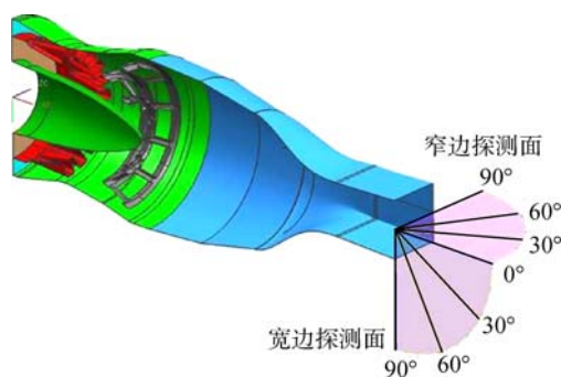
图 4 探测面方位角示意图
