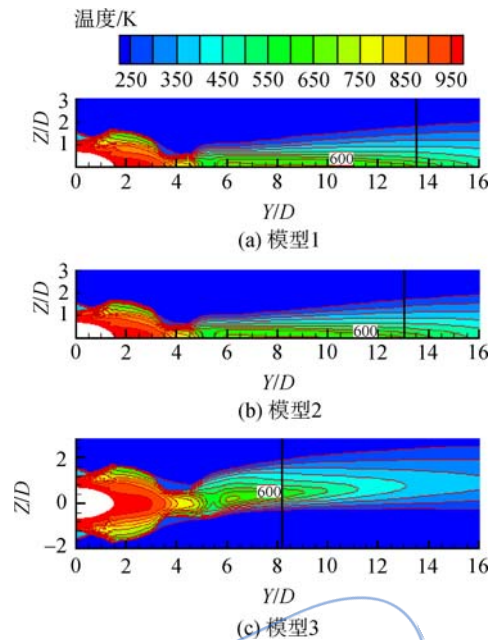
图6 喷管窄边对称面射流温度分布
